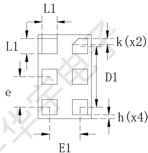
背视图
