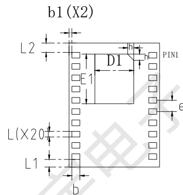
背视图
