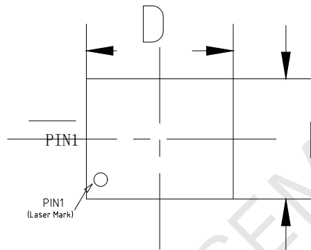
正视图
