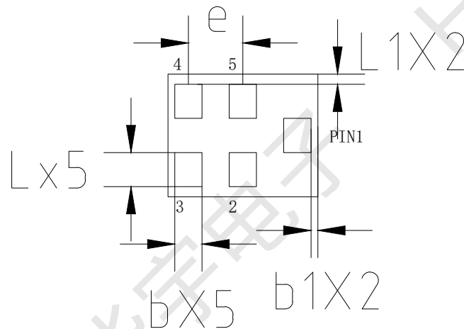
背视图
