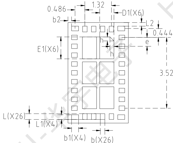
背视图
