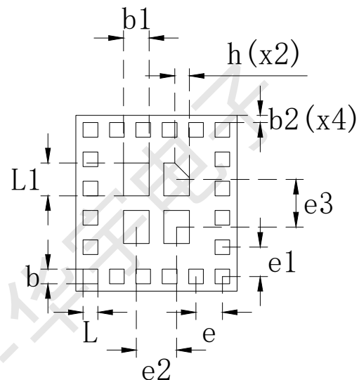
背视图
