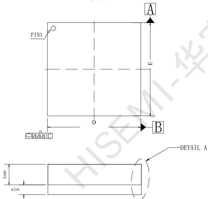
正视图
