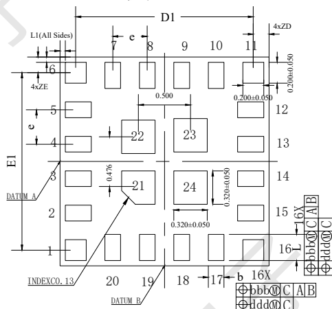
背视图
