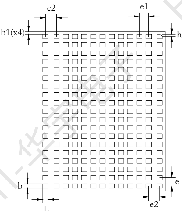
背视图
