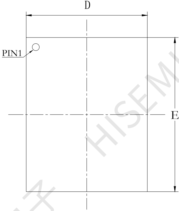
正视图
