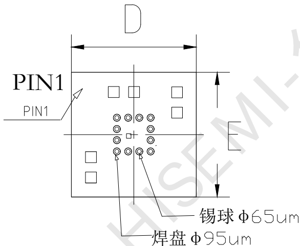
TOP VIEW 正视图
