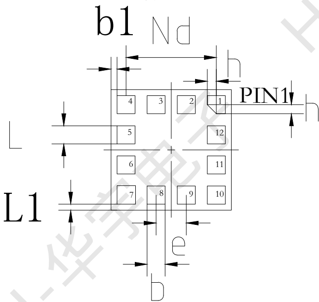
BOTTOM VIEW 背视图
