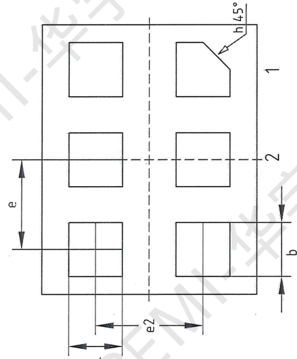
BOTTOM VIEW 背视图
