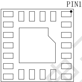
底部示意图
